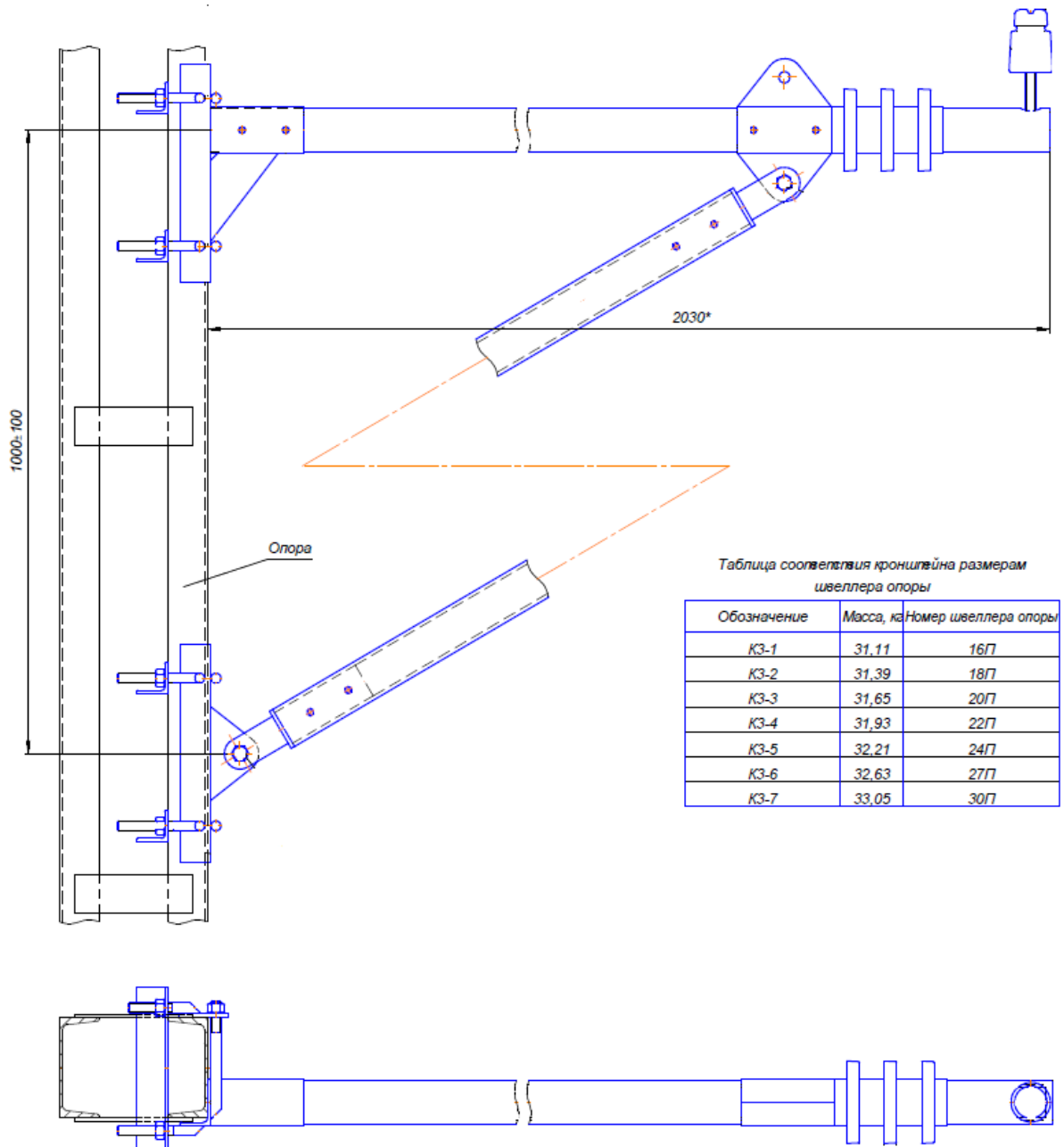
Рис.1 Диэлектрические кронштейны ДК-В-1У
